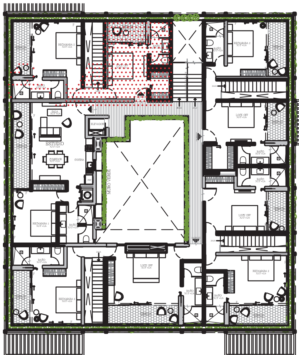
PLANTA NIVEL 1
