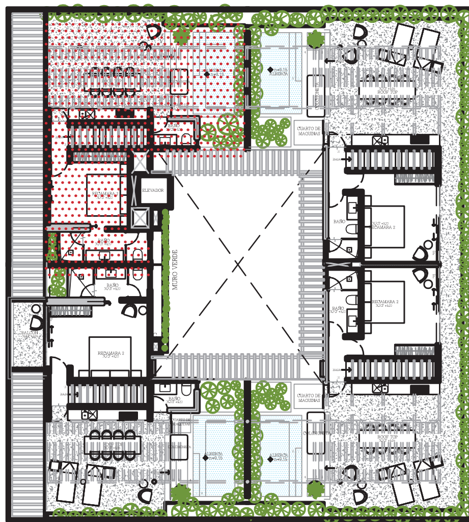
PLANTA NIVEL PH
