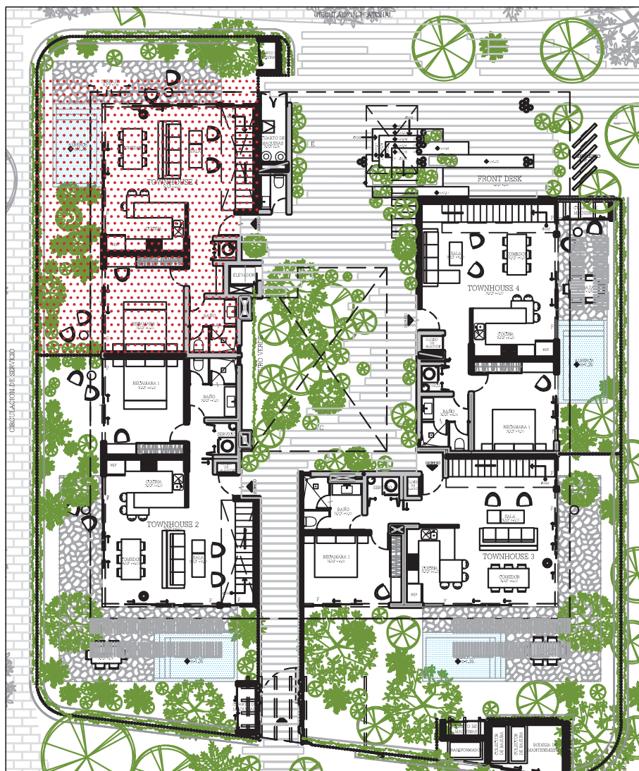
PLANTA BAJA
