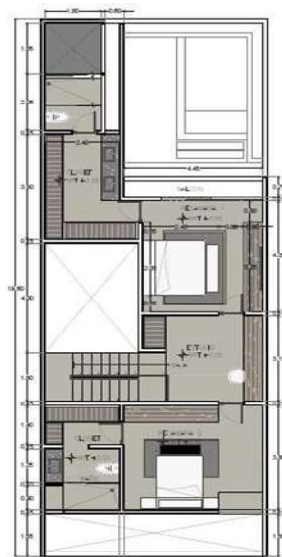
PLANTA ALTA ESCALA 1:100
