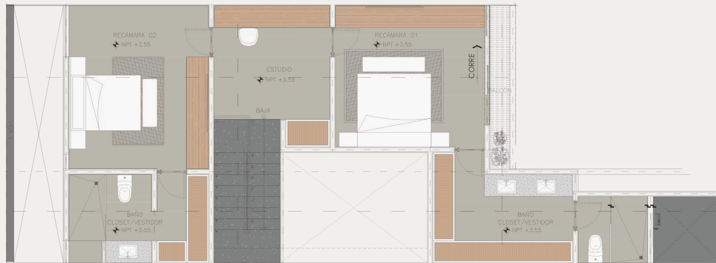
PLANTA ALTA
