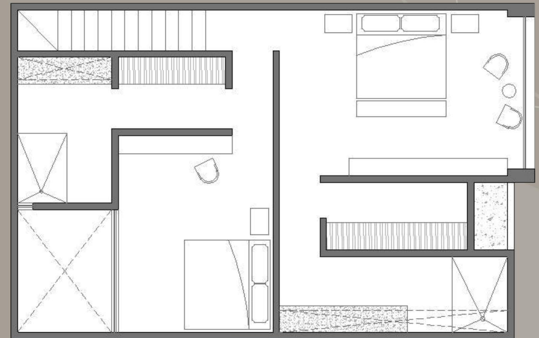
PLANTA ALTA
