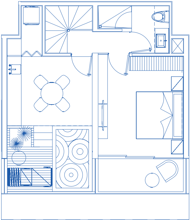
Planta Alta
