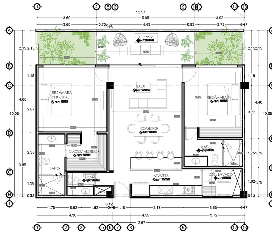
PLANTA ARQUITECTÓNICA
