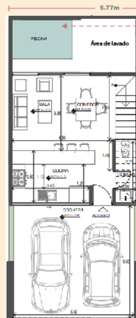
Planta baja
