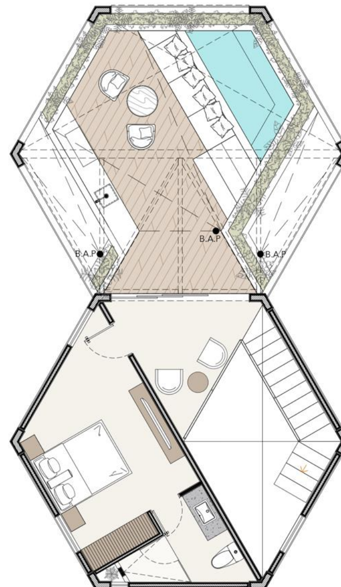
PLANTA ALTA
