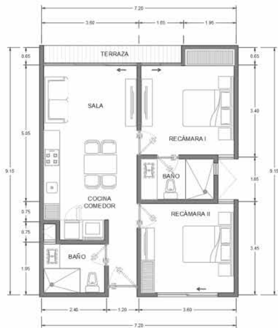
DEPARTAMENTOS TIPO 2 (2 REC) 66.87 M2
