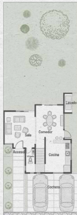
Planta baja
