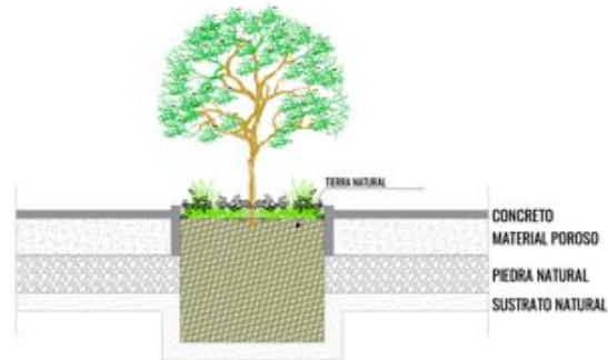
Detalle de Poceta
