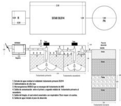
Detalle de SITAR DLD14 con pozo de absorción (Sin escala)
